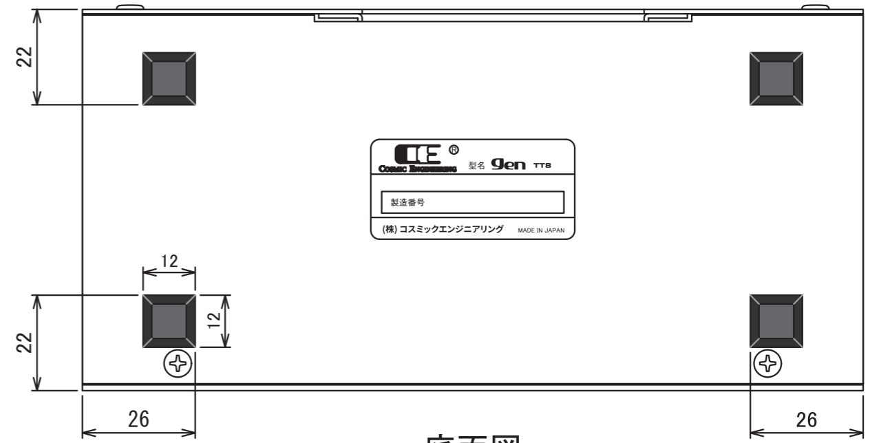
-底面図-
